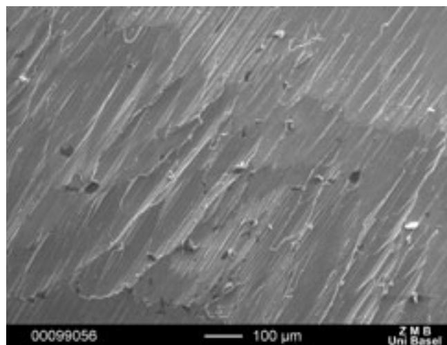
Abb. 7 REM-Aufnahme des bearbeiteten Implantates mit dem Instrument Nr. 6 (100-fache Vergrößerung)
